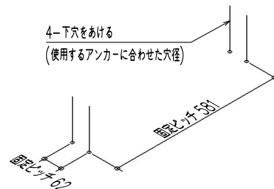
〈図1〉アンカーの下穴あけ
