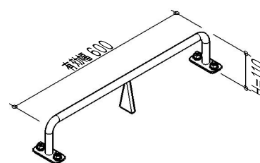
〈図3〉製品の寸法図
