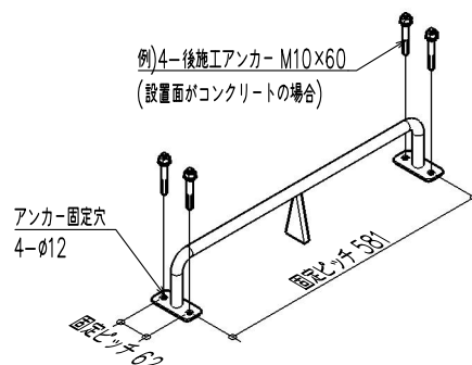
〈図2〉アンカーの固定
