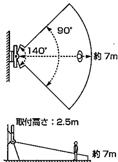
■検知エリア図（2.5m取付時）
