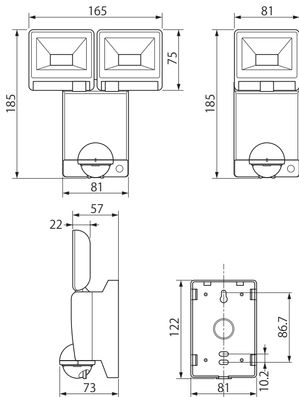
■外形寸法図
