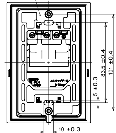
裏面 取付寸法
