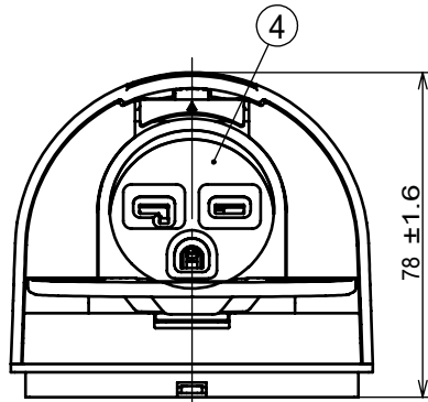
コンセントカバーを開いた状態
