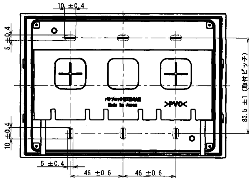
裏面 取付寸法
