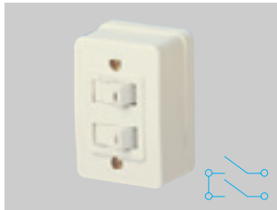
㊦WS3900W 希望小売価格 760円 税抜 2連タンブラスイッチ(ハイ角連用) 10A300V
