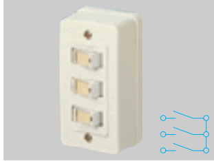
㊦WS3910W 希望小売価格 1,300円 税抜 3連タンブラスイッチ(カード付) 10A300V
