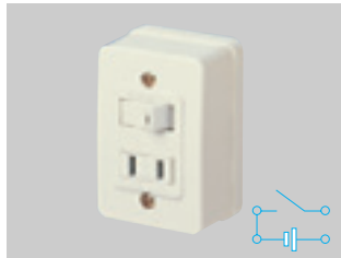
㊦WS3901W 希望小売価格 700円 税抜 コンセント付タンブラスイッチ(ハイ角連用) スイッチ10A300V コンセント15A125V
