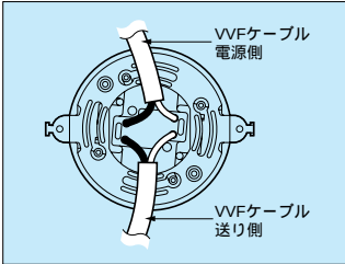
●WG6420WK 希望小売価格 820円 税抜 コンセント付引掛埋込ローゼット(ミルキーホワイト) (送り端子付) 6A125V
