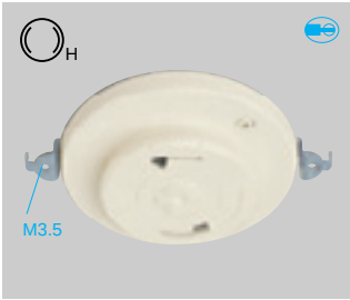
●WG6005W 希望小売価格 500円 税抜 フル引掛ローゼット(露出・埋込両用) (ミルキーホワイト) (送り端子付) 6A 125V ●WG6005A 希望小売価格 500円 税抜 チョコ色もあります。
