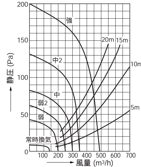
静圧-風量特性 (150)
