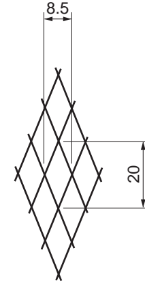
金網拡大図
