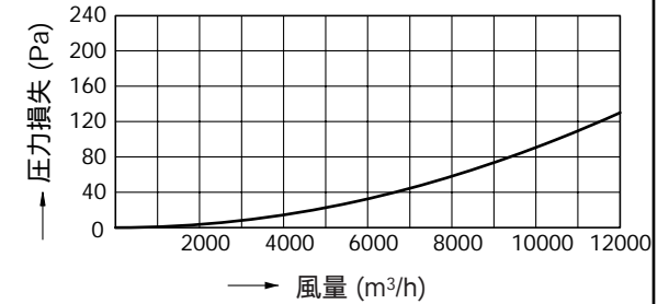
圧力損失曲線 (VP-61-S 2 ) 圧力損失係数 = 排気3.6
