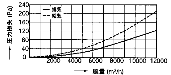
■ 圧力損失曲線：給気 (VP-60MT 2 ) ※ 圧力損失係数 ζ = 排気3.5、給気5.7
