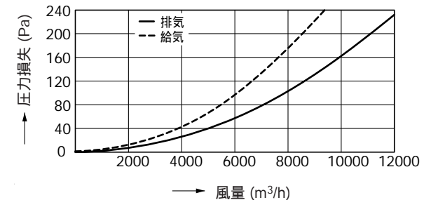
圧力損失曲線：給気（VP-50MT 2 ） 圧力損失係数 = 排気3.3、給気5.5
