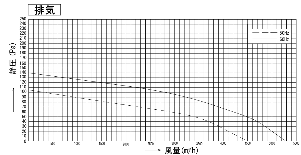
■ 静圧 — 風量特性
