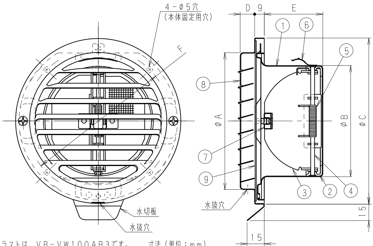
※イラストは、VB-VW100AB3です。 寸法 (単位: mm)
