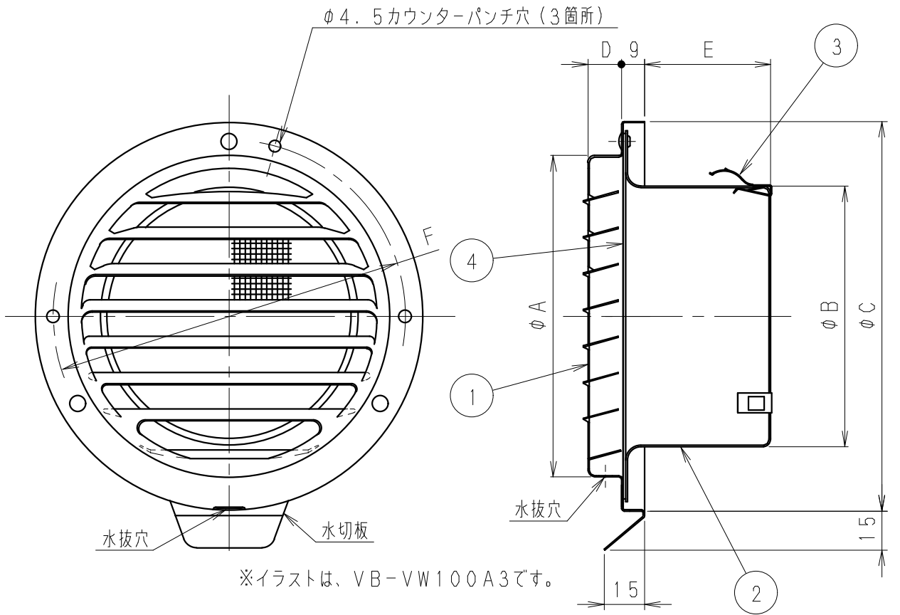
寸法 (単位: mm)
