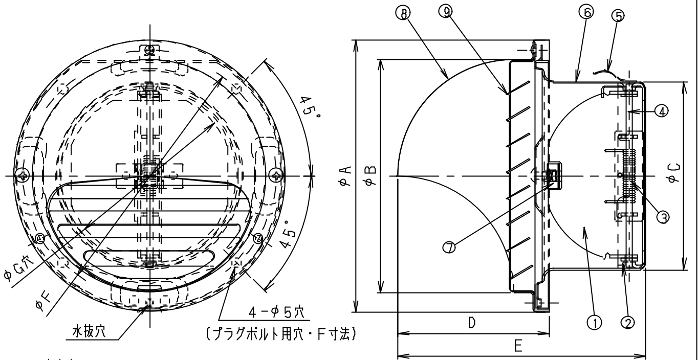
■寸法表
