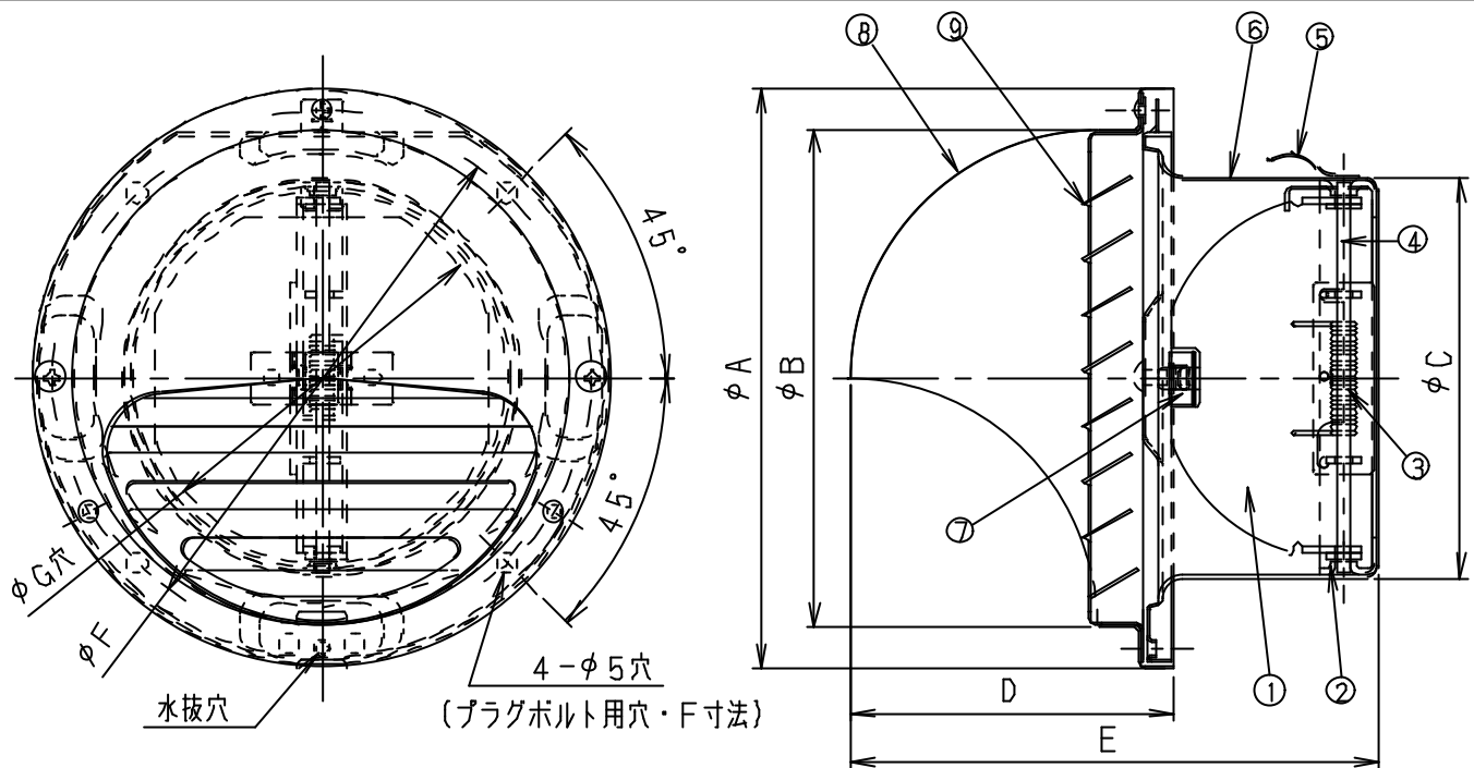
■寸法表
