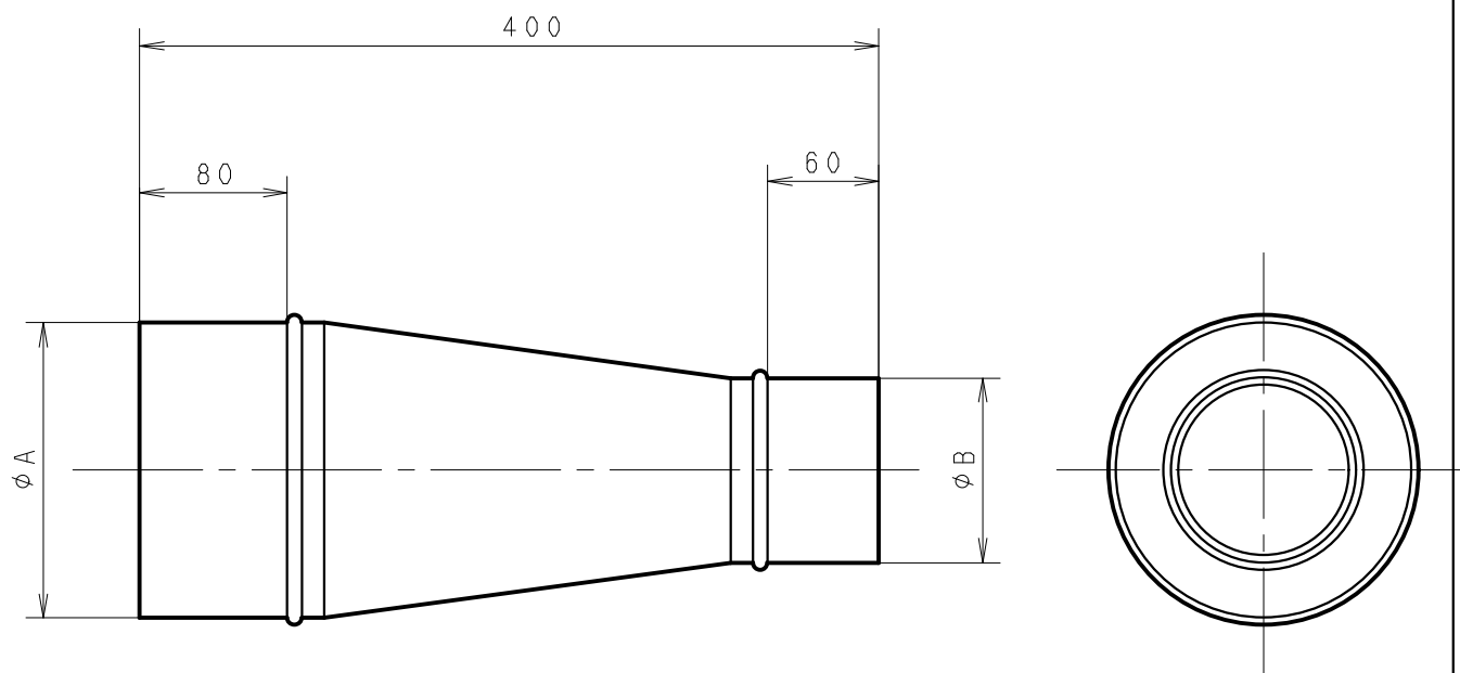
■ 寸法表
