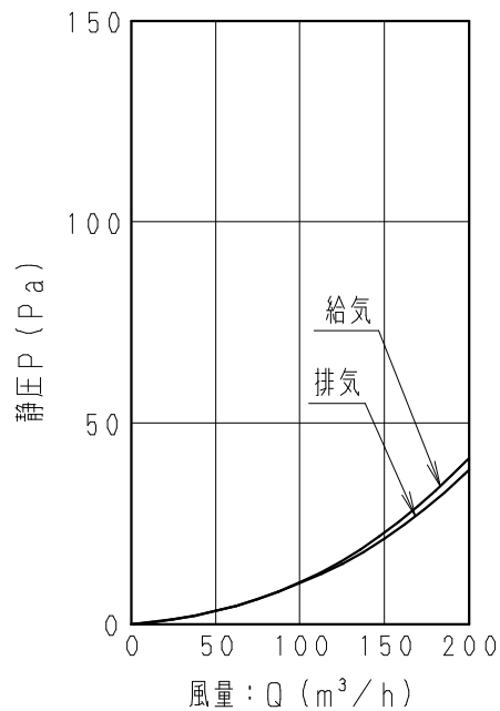
■ 抵抗損失曲線
