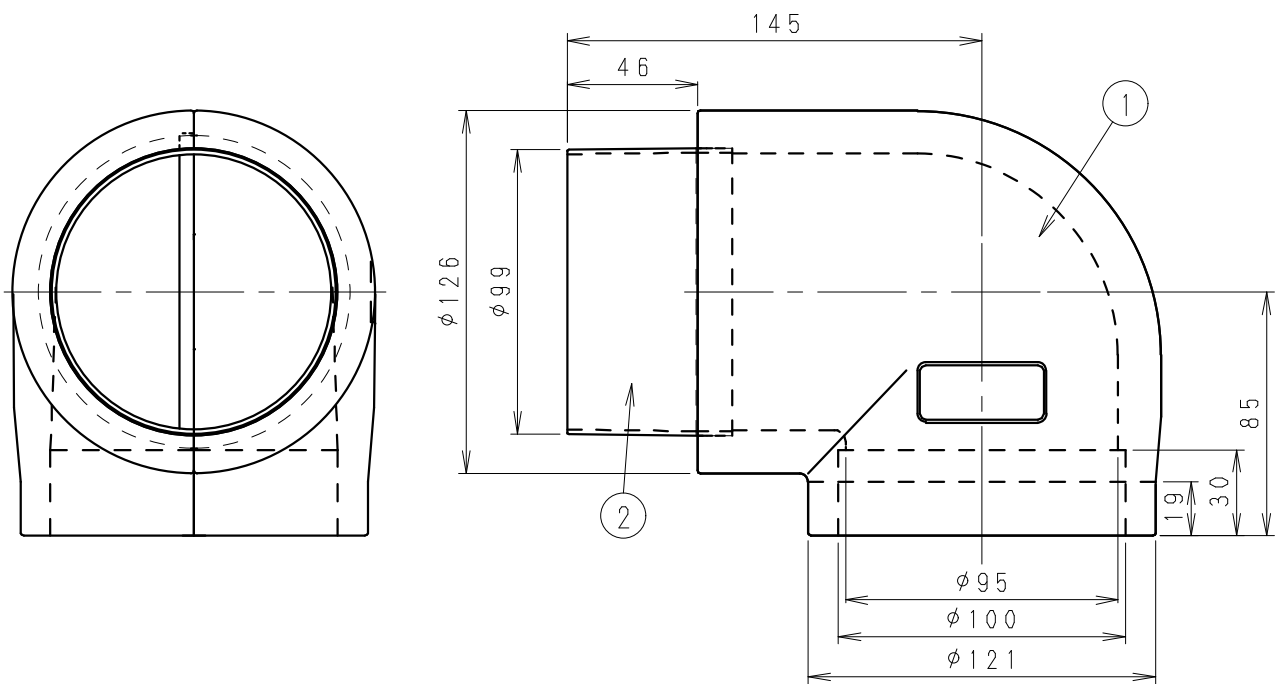
■ 部品表
