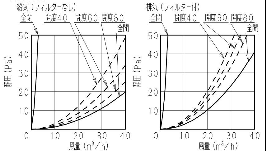
■抵抗損失曲線
