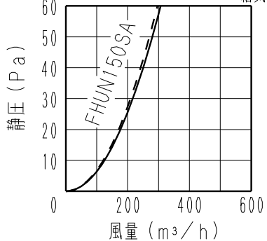
■ 抵抗損失曲線
