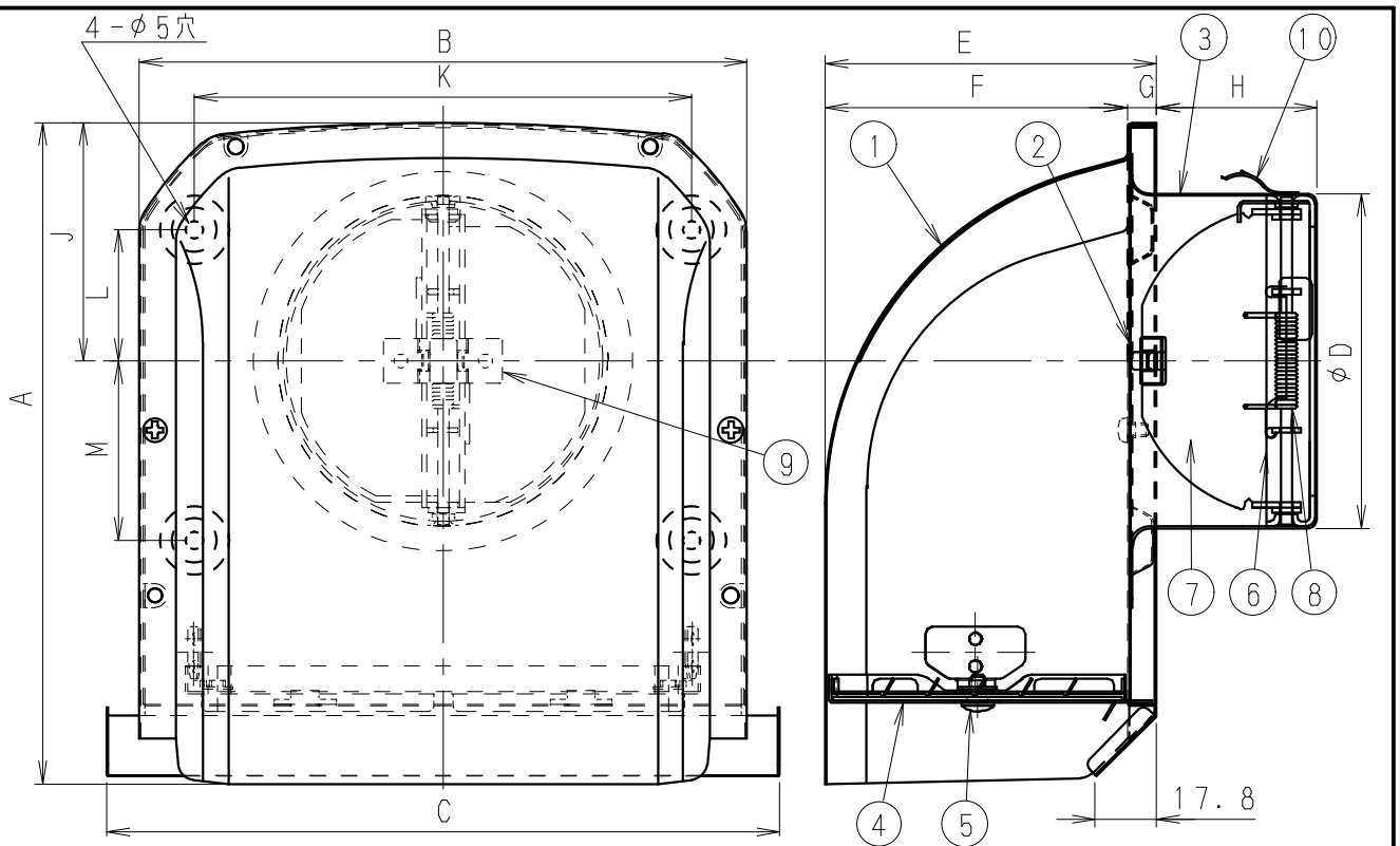
■寸法表
