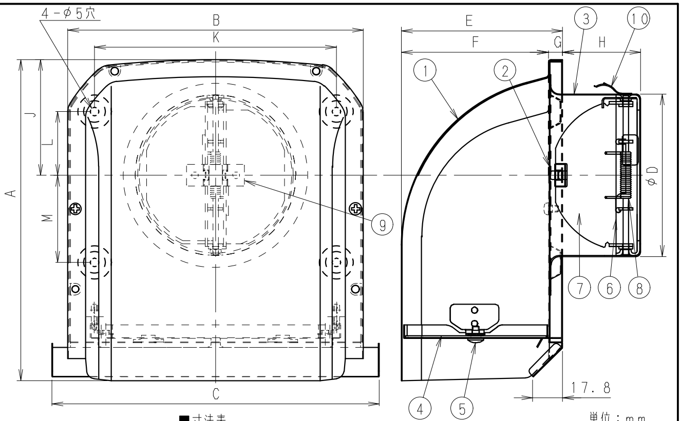
■寸法表
