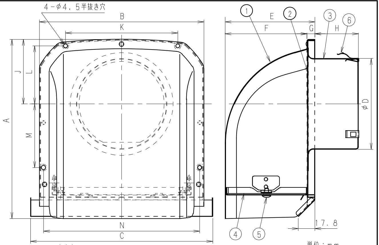
■寸法表
