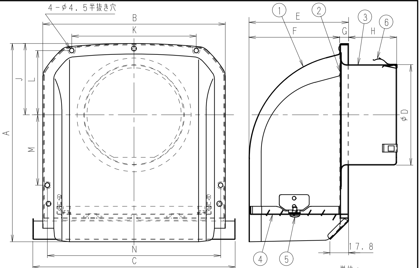
■ 寸法表
