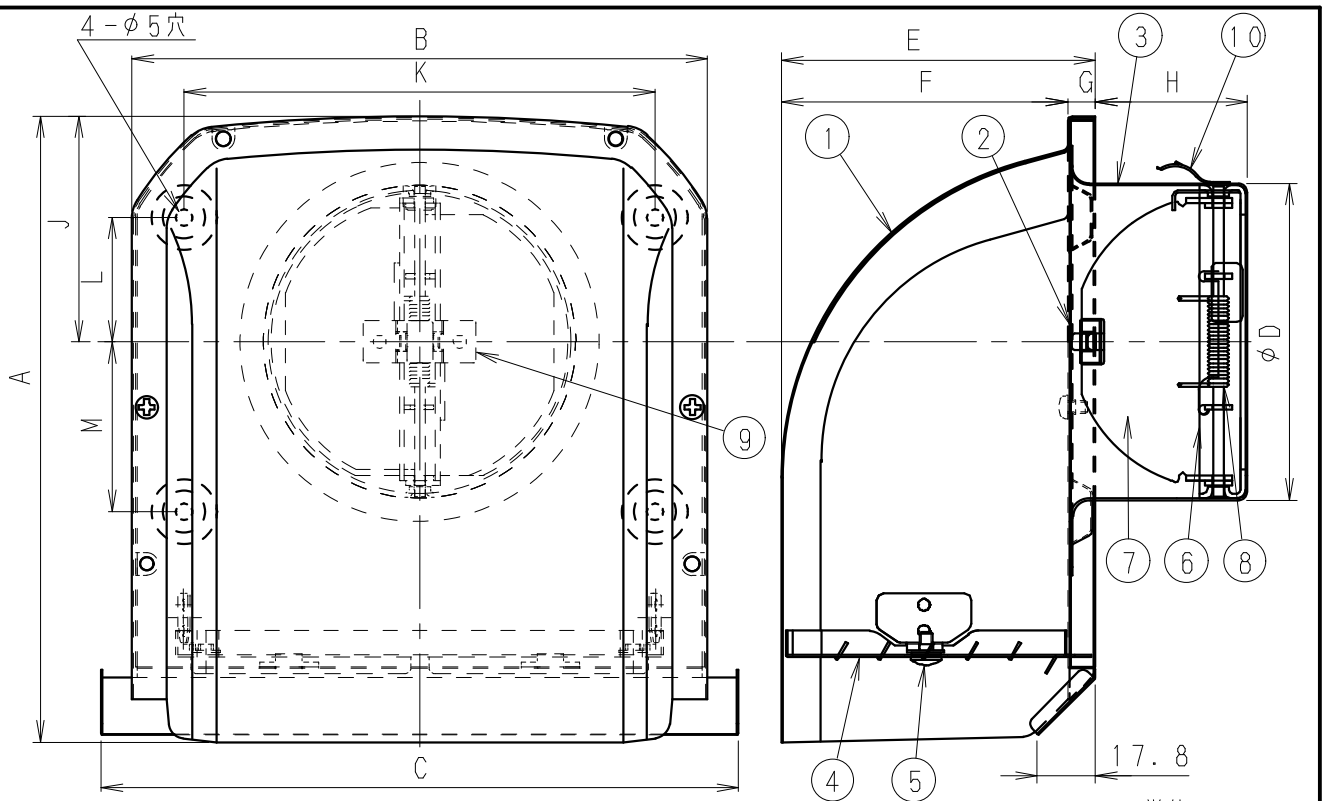
■寸法表
