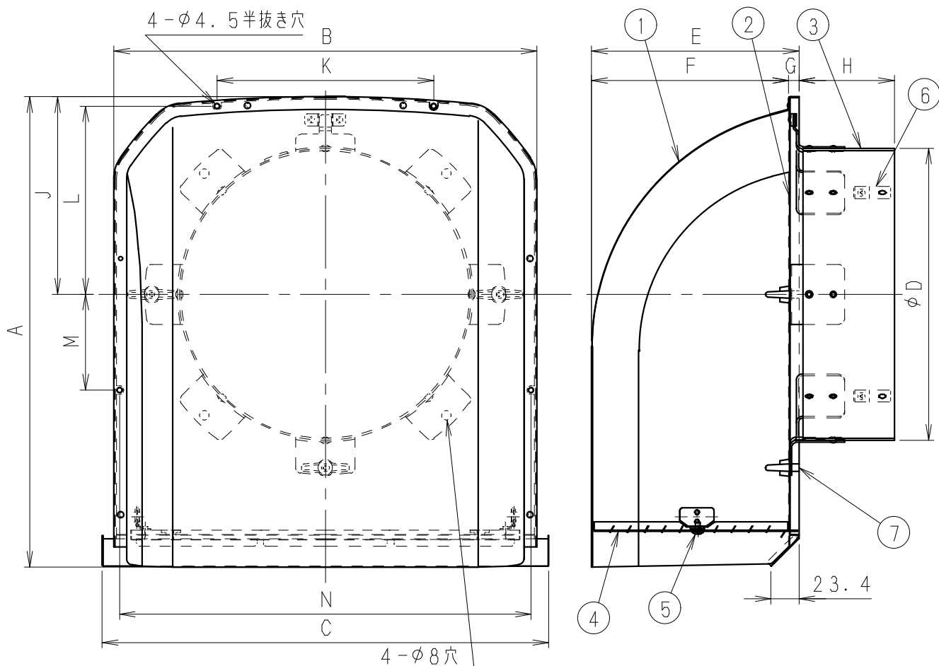
■ 寸法表
