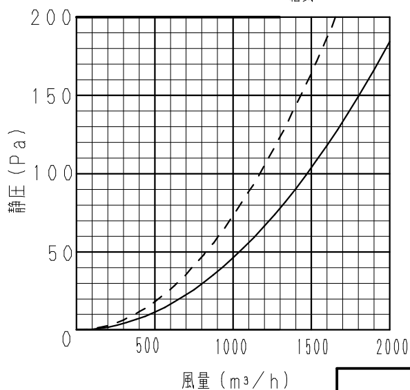
■ 抵抗損失曲線
