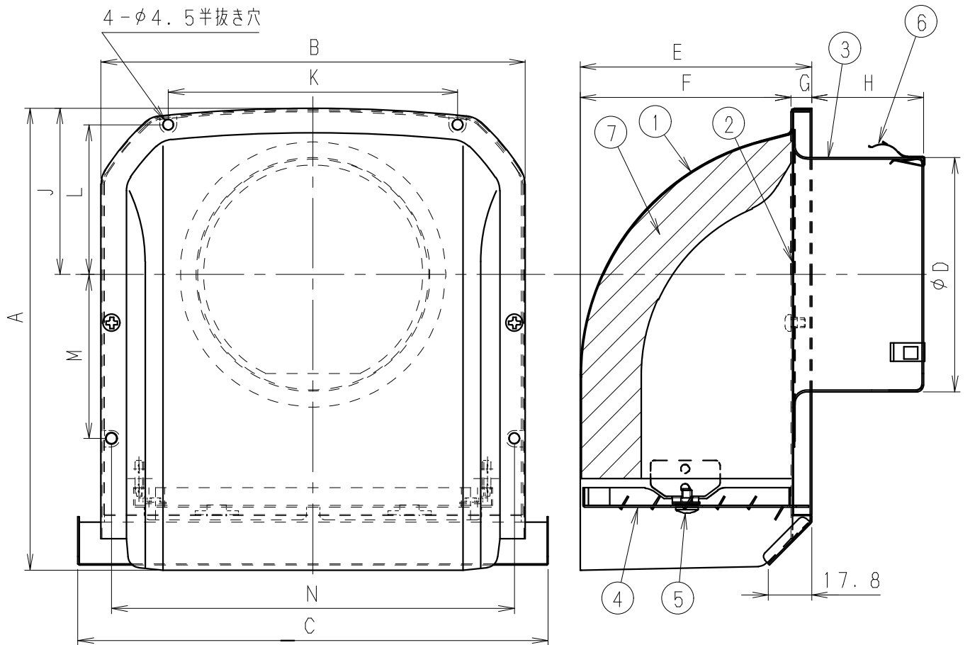
■ 寸法表
