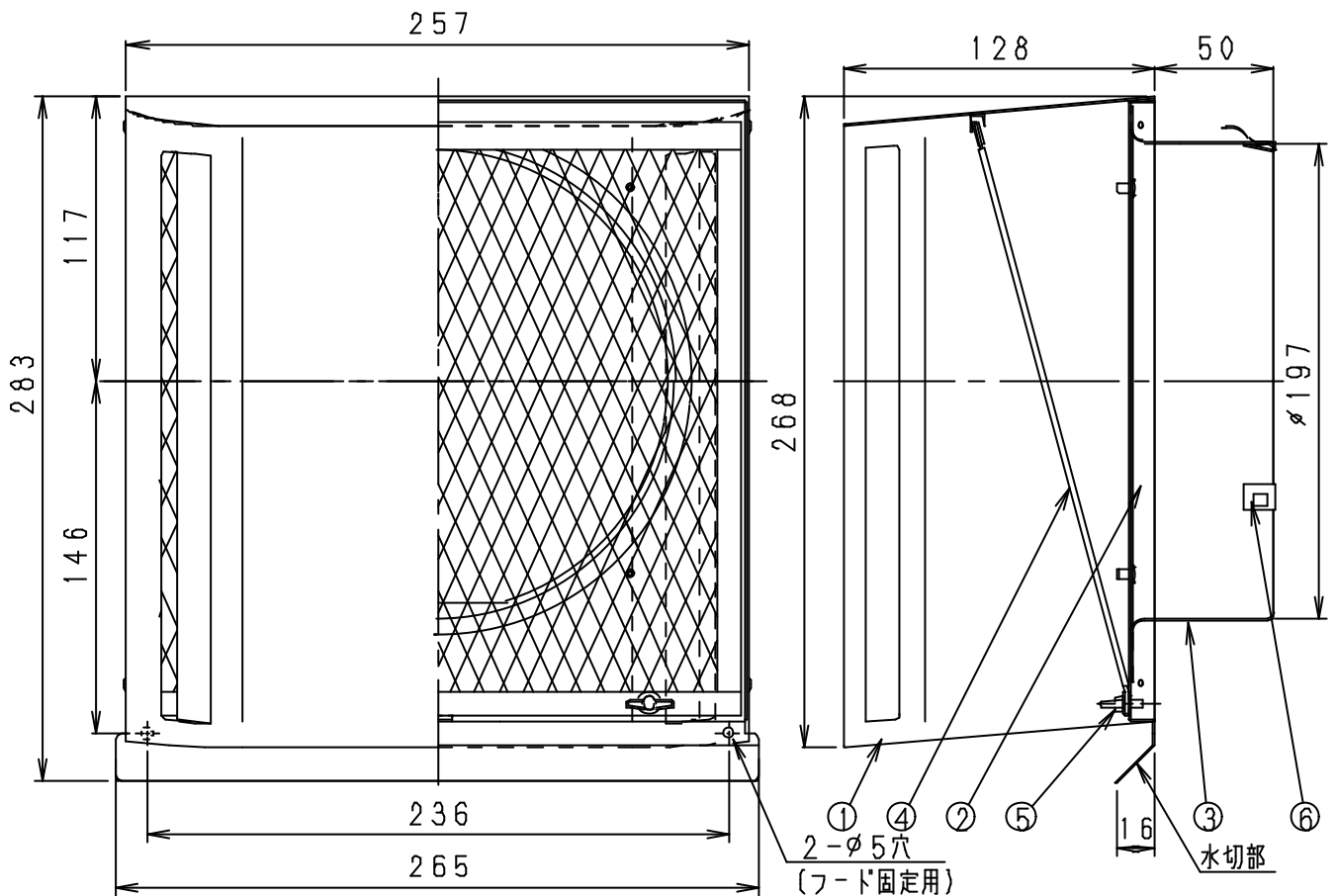
寸法 (単位: mm)
