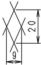
防鳥網寸法
