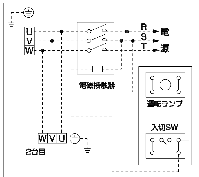
結線例
