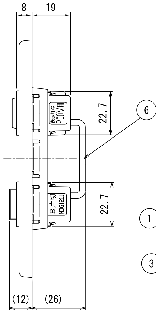
結線例
