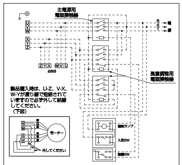
結線例
