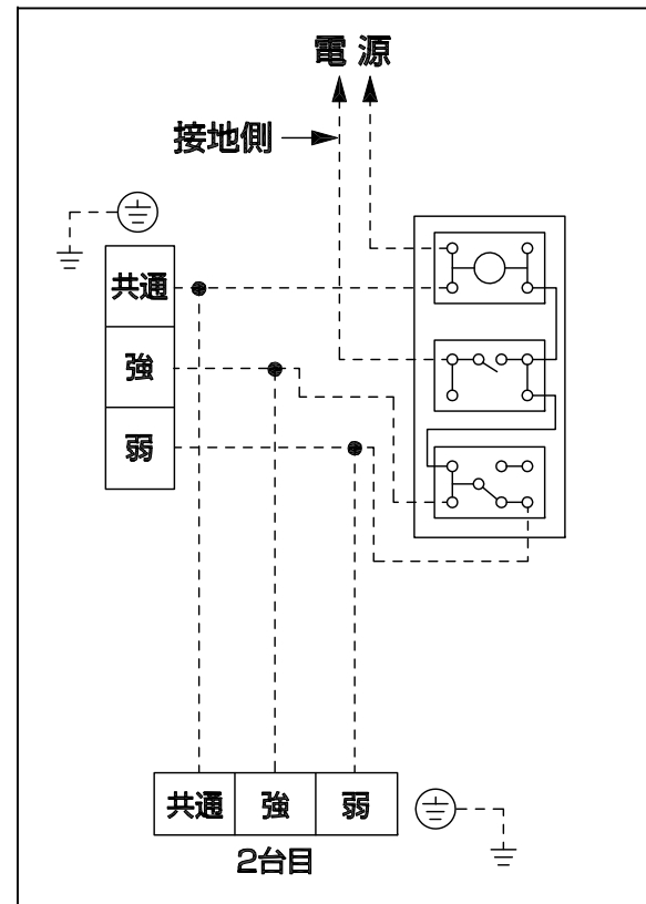
結線例
