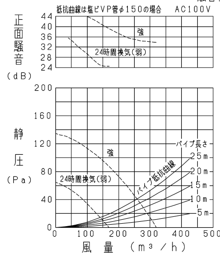
VD-18ZLC 12 -IN/P-Q・騒音特性
