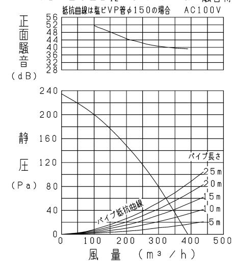
VD-20ZB 12 -IN/P-Q・騒音特性
