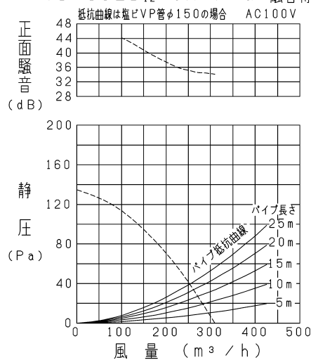
VD-18ZB 12 -IN/P-Q・騒音特性
