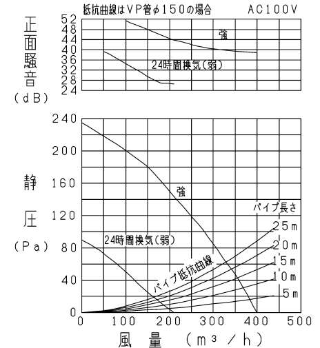
VD-20ZLC 12 -IN/P-Q・騒音特性
