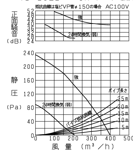
VD-20ZLC 9 -IN/P-Q・騒音特性
