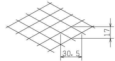
■ 金網拡大図
