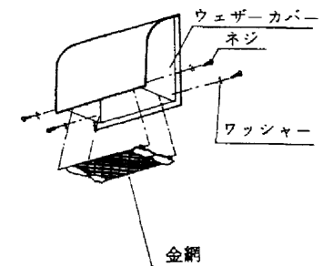
取付図
