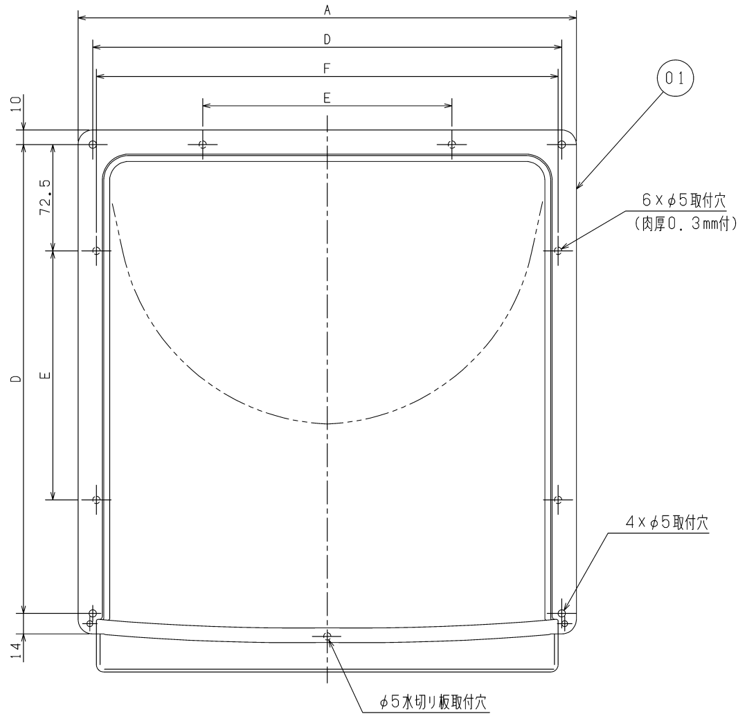
■変化寸法表
