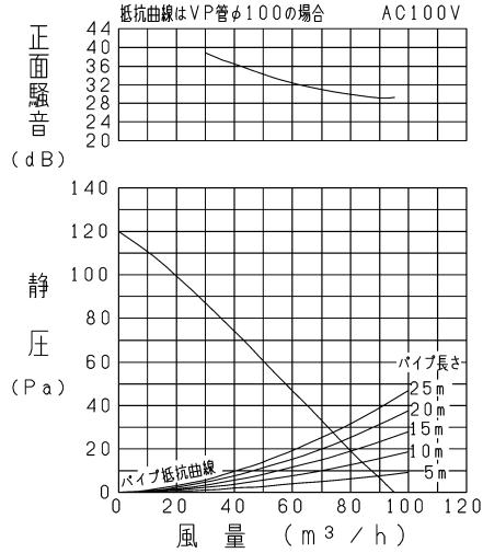
VD-10Z 12 -IN/P-Q・騒音特性
