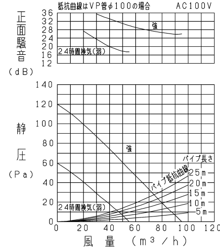
VD-10ZLC 12 -IN/P-Q・騒音特性
