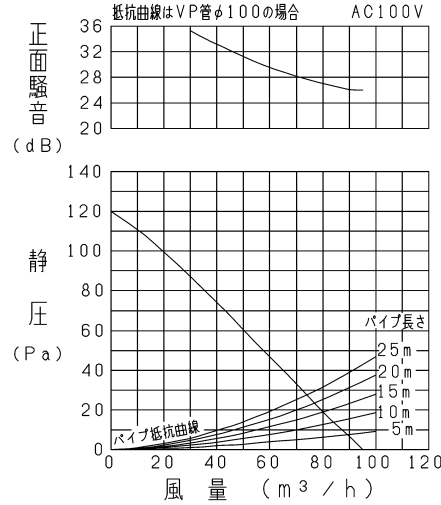
VD-10ZC 12 -IN/P-Q・騒音特性
