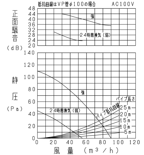
VD-10ZLUC 2 -IN/P-Q・騒音特性
