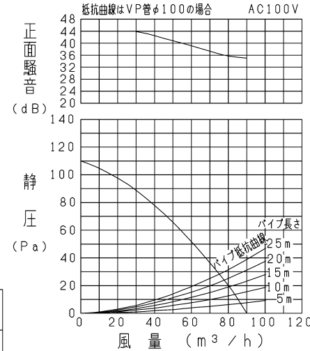
VD-10ZUC 2 -IN/P-Q・騒音特性
