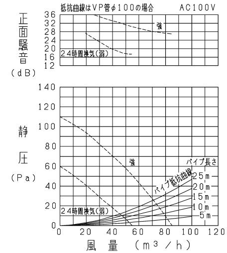
VD-10ZLC 12 -IN/P-Q・騒音特性
