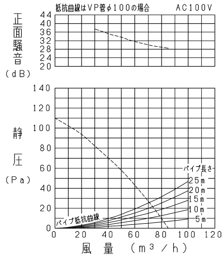
VD-10Z 12 -IN/P-Q・騒音特性
