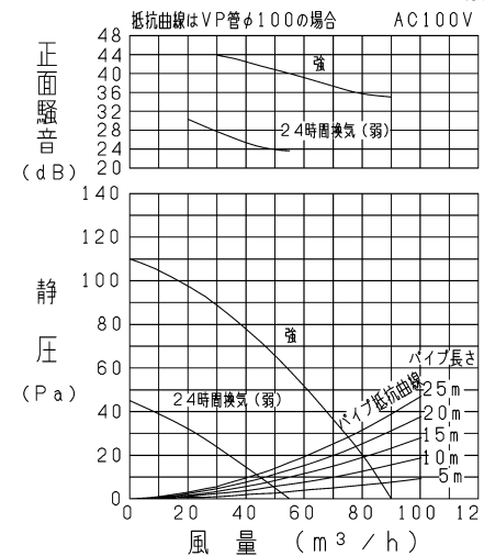
VD-10ZLUC 2 -IN/P-Q・騒音特性
