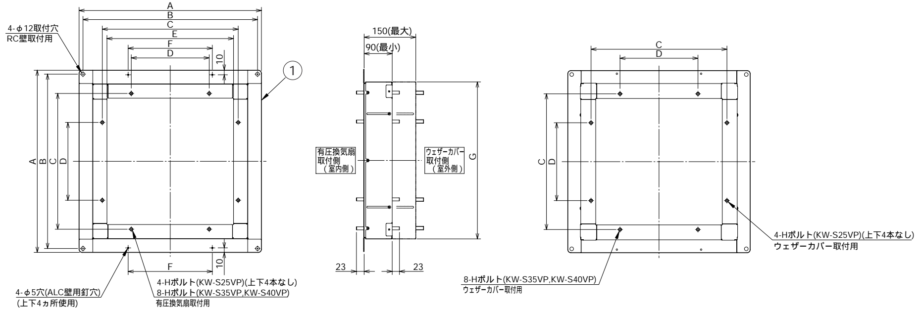
寸法表
