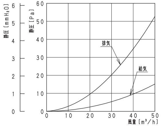
■ 抵抗損失曲線
