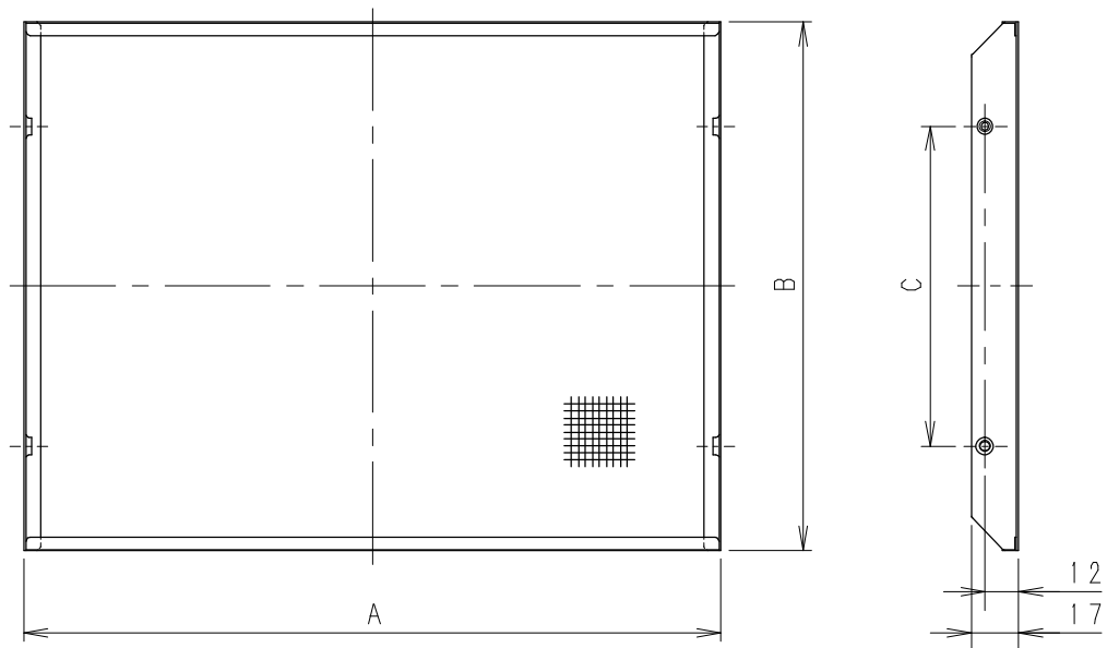
■寸法表
