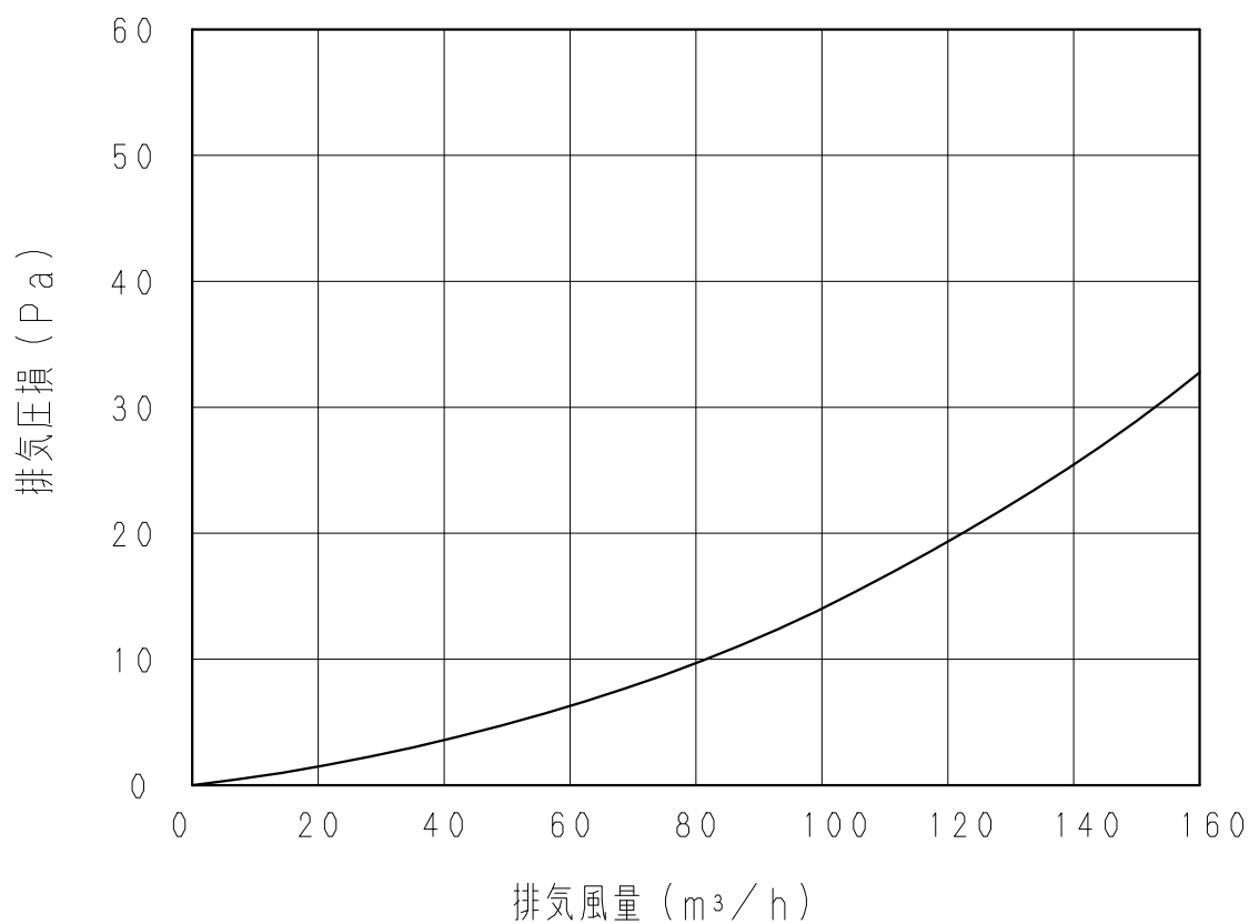
■ 抵抗損失曲線（排気圧損）
