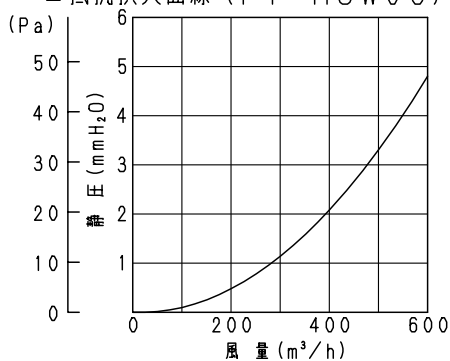
■抵抗損失曲線（FY-MSW04）
