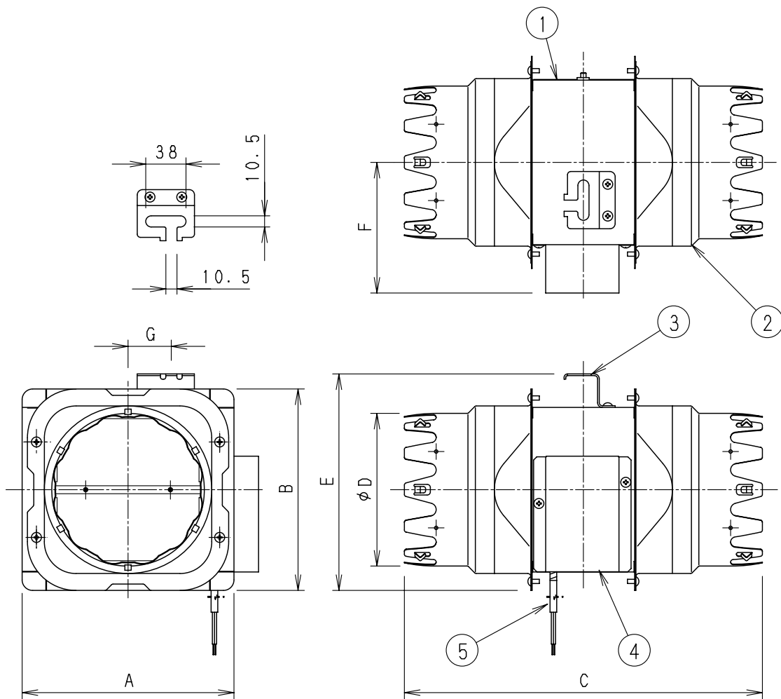
■寸法表（低圧損）
