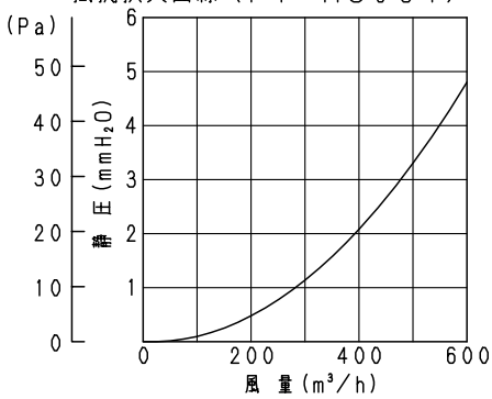
■ 抵抗損失曲線 (FY-MS044)
