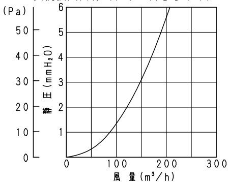
■ 抵抗損失曲線 (FY-MS044)
