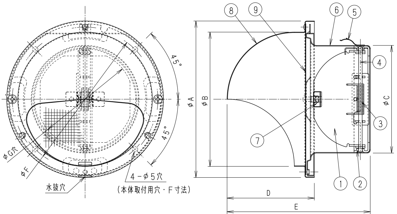
■寸法表
