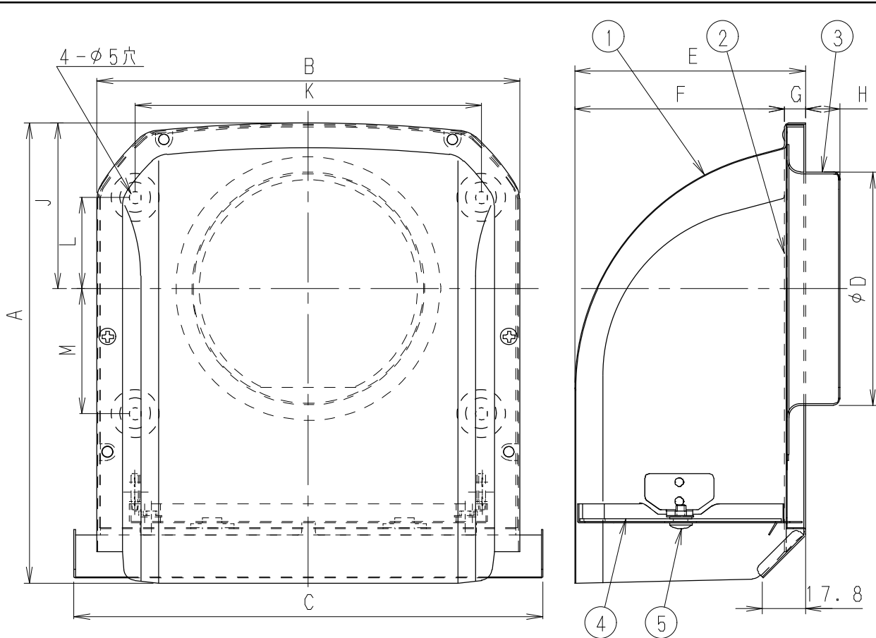
■ 寸法表
